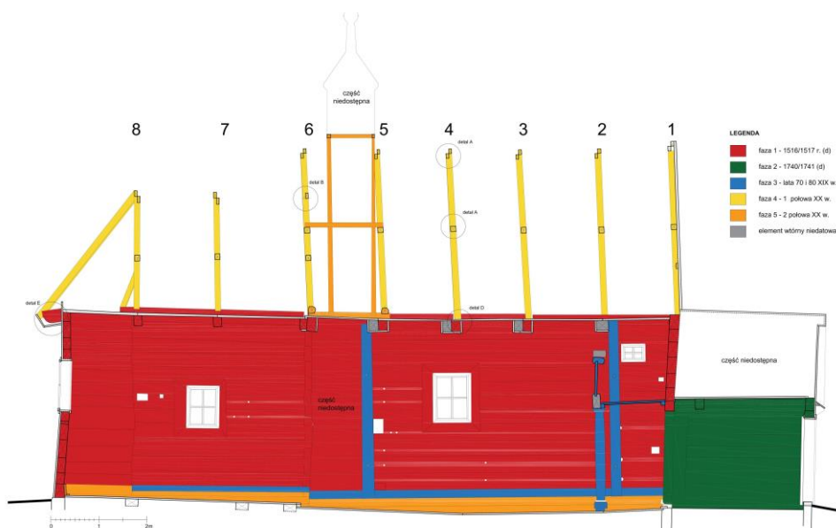
Kaplica cmentarna w Szczercowie – rozwarstwienie chronologiczne, skala 1-20, oprac. dr M. Prarat.
